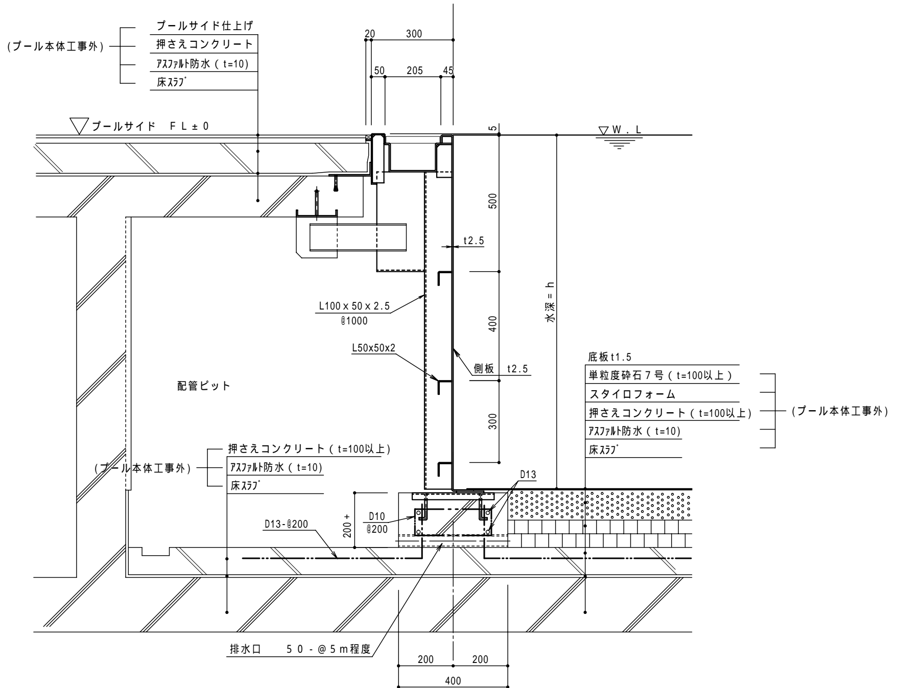
塗装 (無塗装) プール本体断面図
